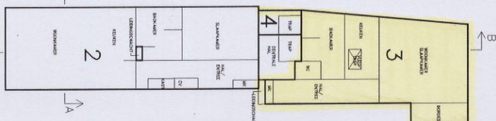
1E VERDIEPING 1:100
