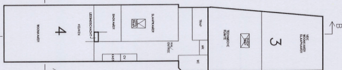
2E VERDIEPING 1:100
